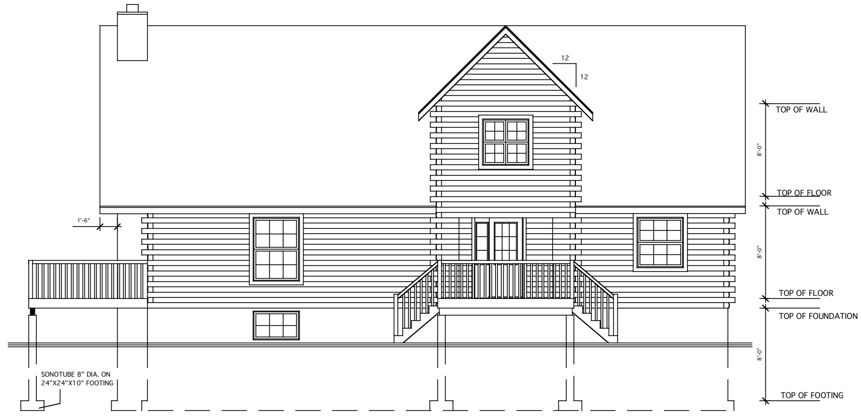
RIGHT ELEVATION
